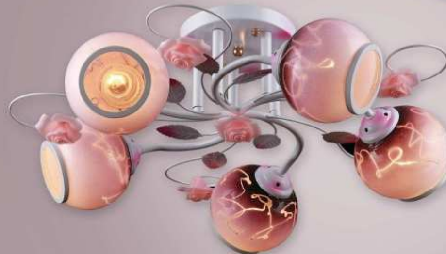
51183-03-C05-WT L: 56cm W: 56cm H: 20cm 1,5 kg Max: 5x40W E-27
